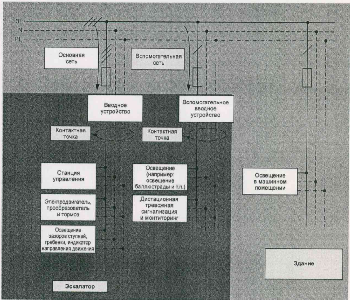
Рисунок А.2 — Подключение средств измерения энергопотребления эскалаторов
