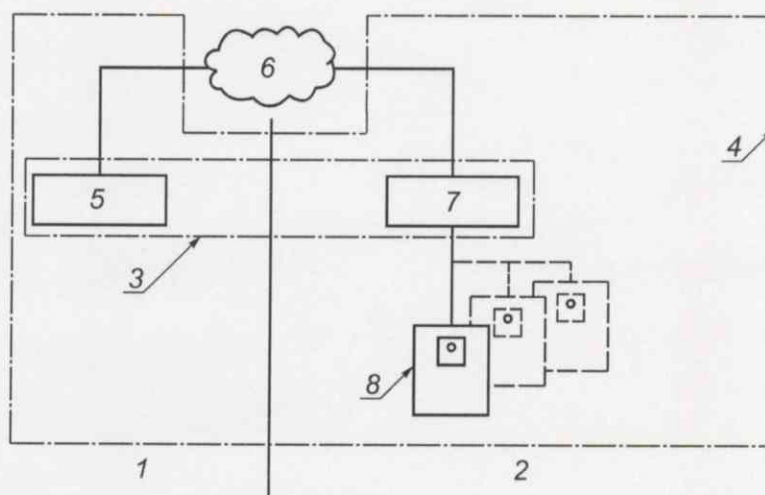
Типовая схема устройства диспетчерского контроля
