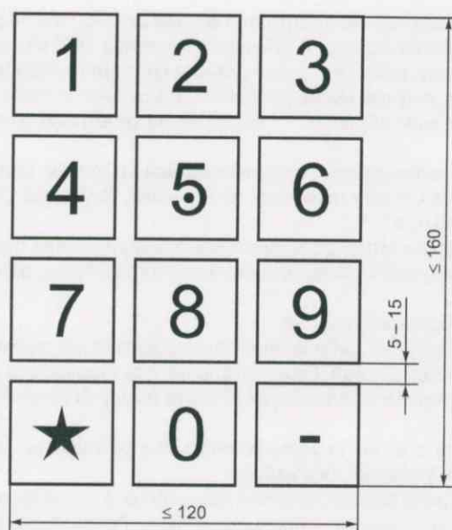
Рисунок 5 — Клавишная панель
