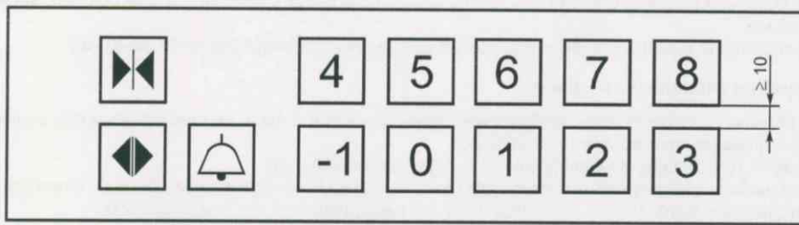
Рисунок В.3 — Пример расположения кнопок в два ряда
