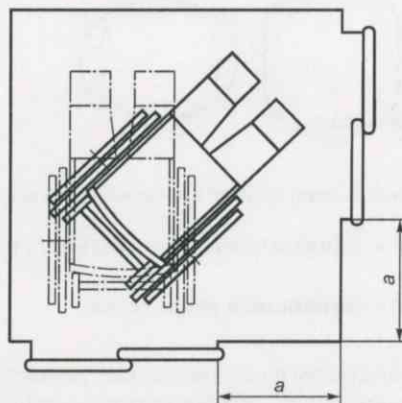
Рисунок 1 — Кабина с дверьми на смежных стенках
